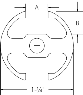
SL-PROFD (2 slots)
