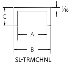
SL-TRMCHNL
