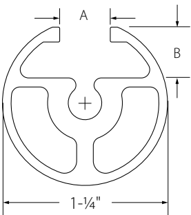
SL-PROF (1 slot)
