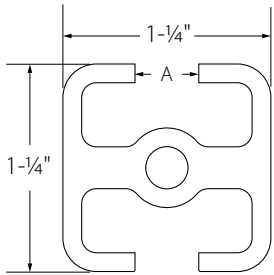
SL-SQPROFD (180° 2-slot)
